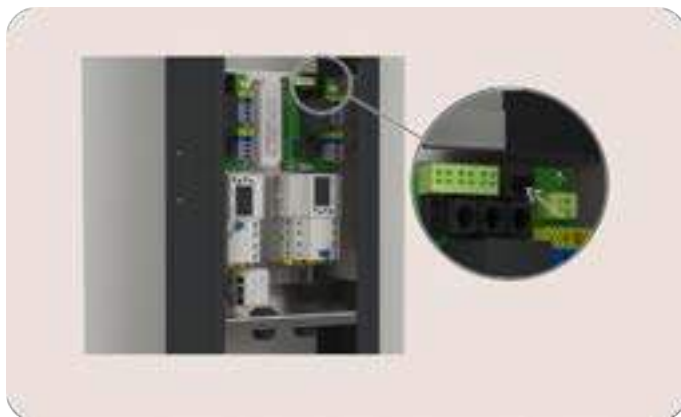
Afbeelding12: aanzicht op de A+B-poort van het relaisbord
