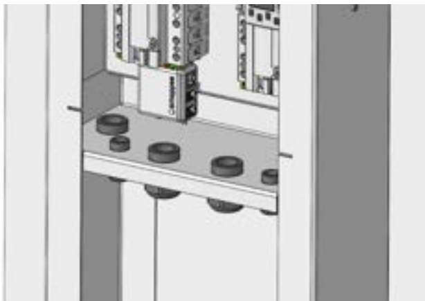
Afbeelding2: aanzicht op de kabeldoorvoer voor de laadkabels
