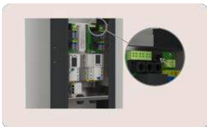
Afbeelding 17: aanzicht op de A+B-poort van het relaisbord
